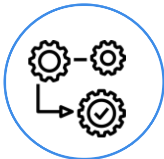
Workflow заказа
